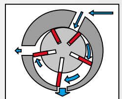
Lamellenmotor
